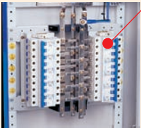
铜排连接构造： 主开关与分支开关 之间采用铜排连接， 不拆卸铜排即可任 意装卸、调整断路 器，维护保养安全、 方便、快捷。
