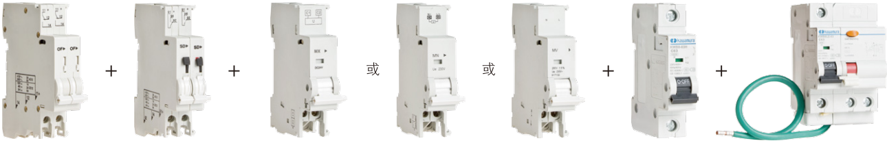
OF+SD/OF 辅助触点 SD 报警触点 MX或MX+OF 分励脱扣器 MV或MNe 电子式欠压脱扣器 MV过压脱扣器 M V +MN 过欠压脱扣器 断路器 漏电附件
