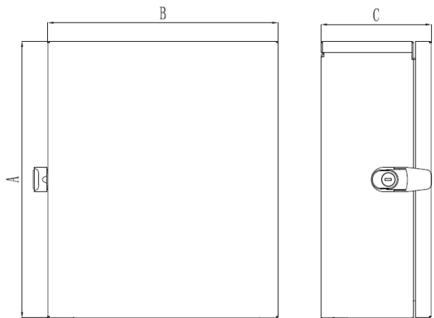
外形图
