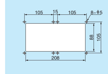
〈安装孔尺寸〉
