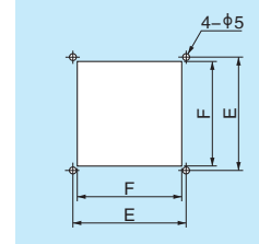
〈安装孔尺寸〉
