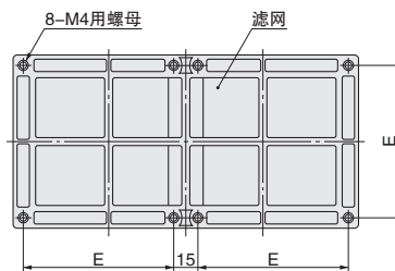
〈安装孔尺寸〉
